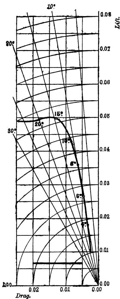
FIG. 1.—Flat plane.
